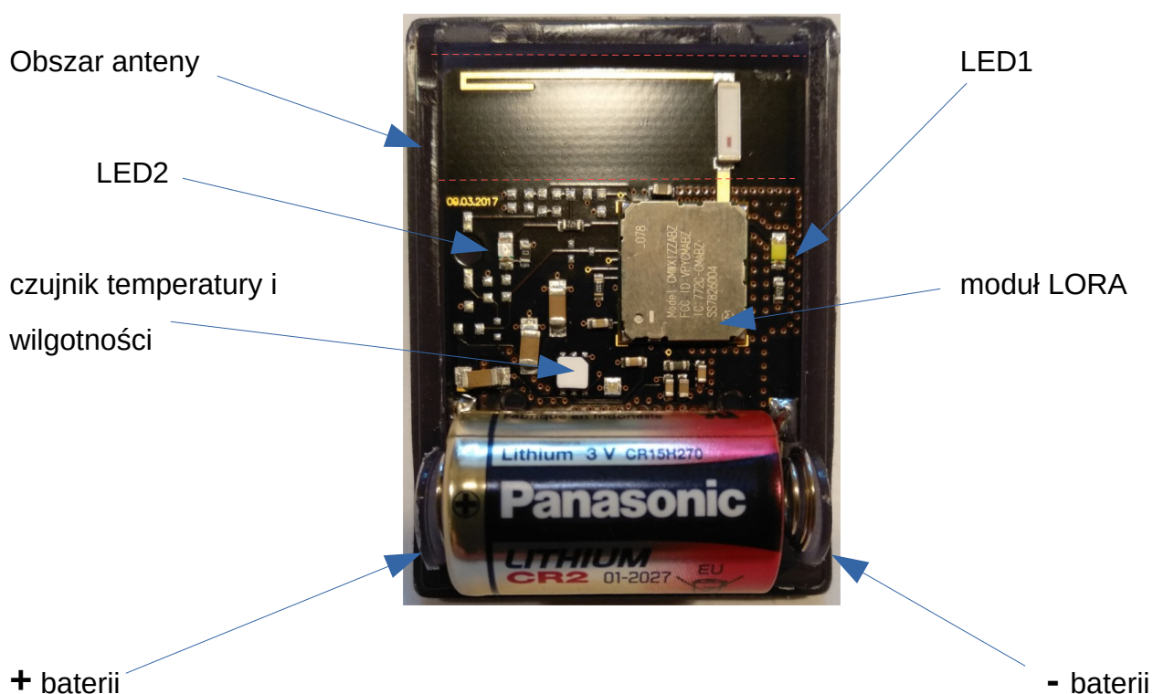
iNode LORA HT – widok po zdjęciu obudowy
